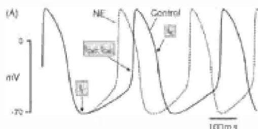
Примечание: Стрелками показаны точки приложения действия I_f , Ca^{2+} T и L типа и отложенного калиевого каналов (ИК) [19]. Рис. 4 Автоматизм синоатриального узла.
